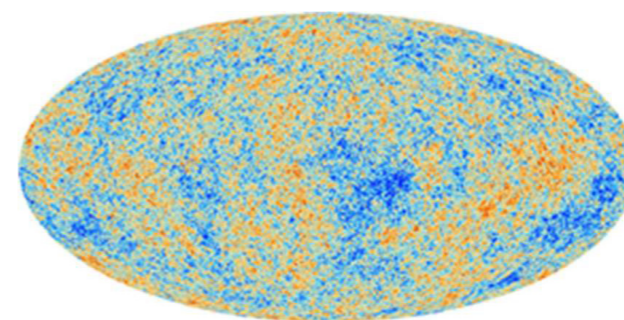
Рисунок.1 – Анизотропия реликтового излучения по телескопу Planck.
